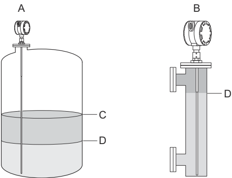
图 11: 界面液位测量
