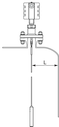
图 14: 可用空间要求
