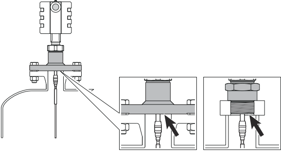
图 9 提供最高过程温度（在法兰式或螺纹式连接件的下方测量）和压力等级：
