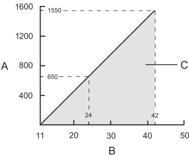
图 5: 非危险安装
