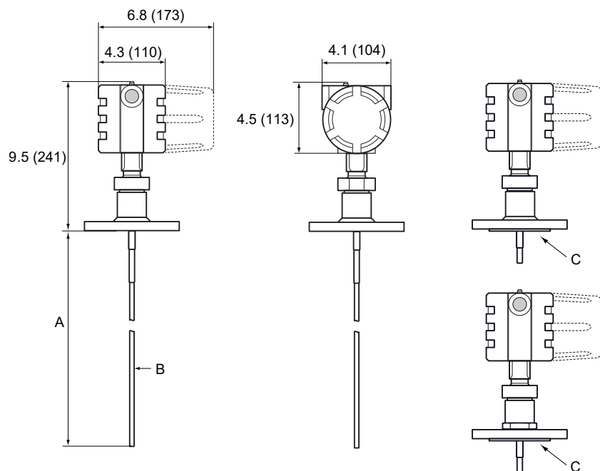
图 22: 采用法兰连接的硬单线导波杆
