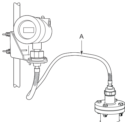
图 12: 远程外壳安装
