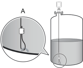
A. 带弓形夹的软单杆导波杆。
