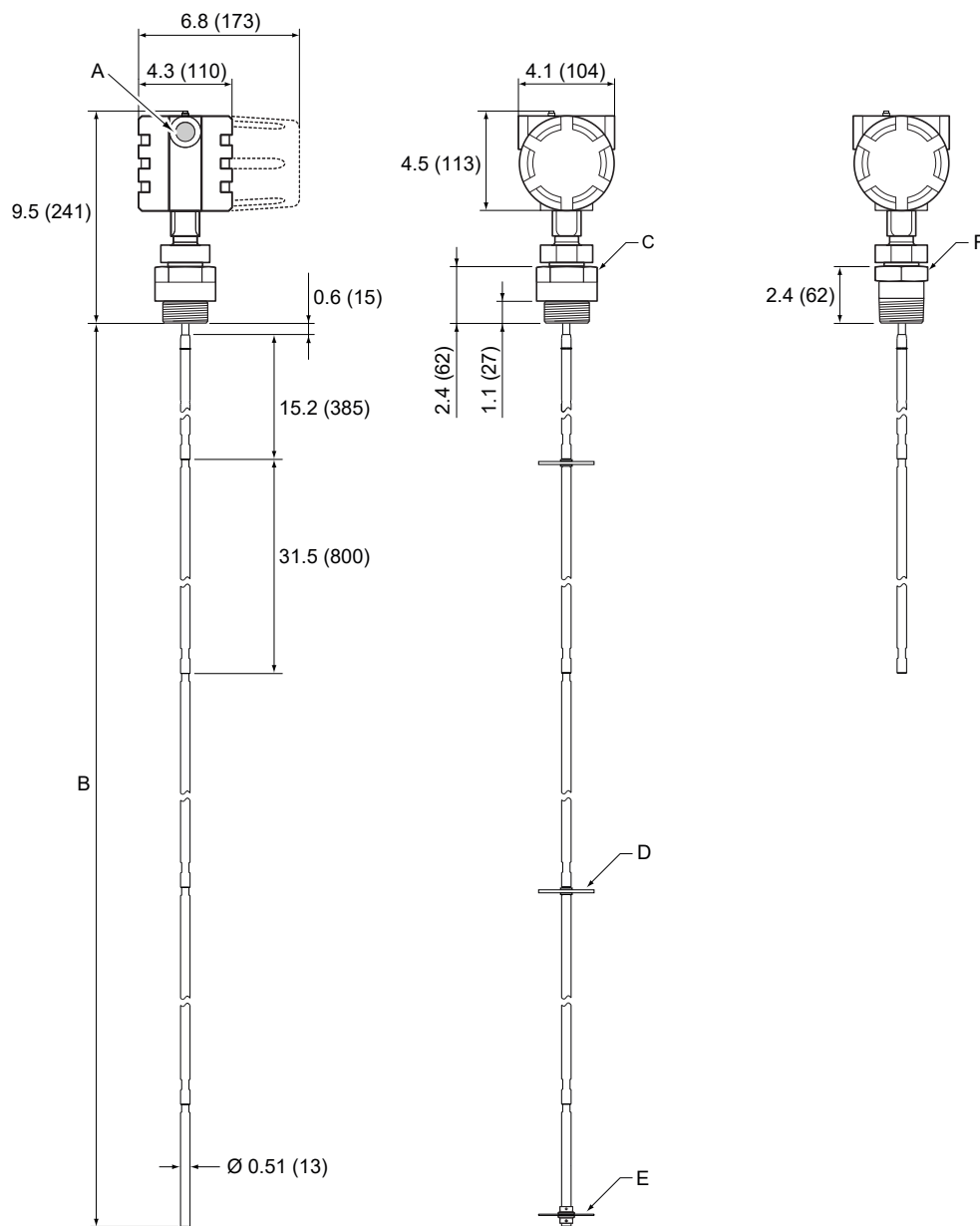
图 25: 采用螺纹连接的分段硬单杆导波杆
