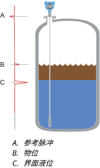
图 1: 测量原理
