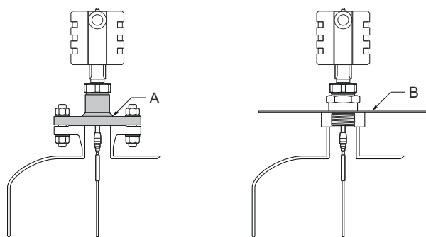
图 20: 安装在非金属储罐中
