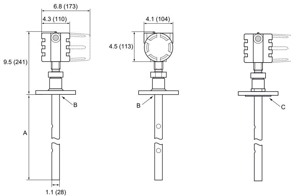
图 28: 采用法兰连接的同轴导波杆
