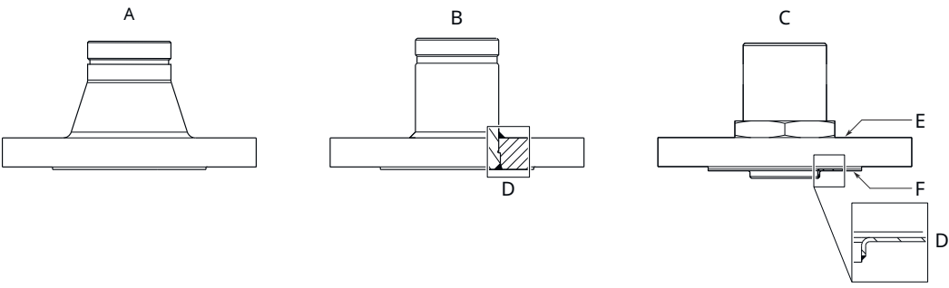
图 32: 法兰连接件
