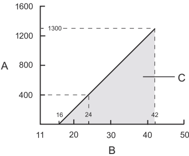
图 7: 防爆/隔爆安装
