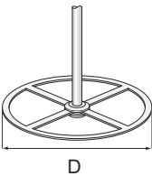
图 17: 定心盘的尺寸 D
