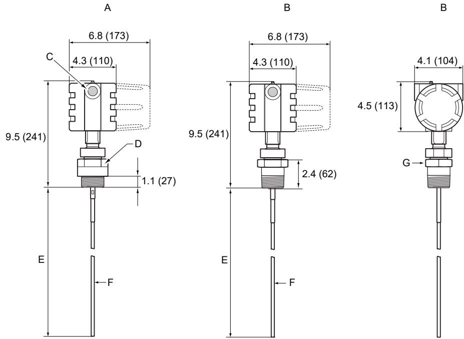
图 23: 采用螺纹连接的硬单线导波杆
