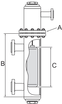
图 16: 现有浮筒旁通管
