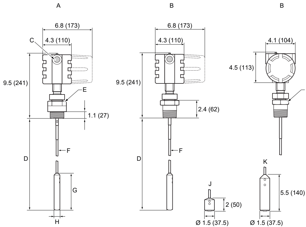
图 27: 采用螺纹连接的软单杆导波杆
