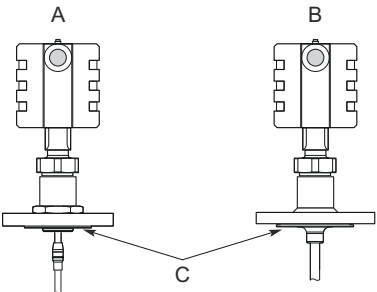
图 10: 保护板
