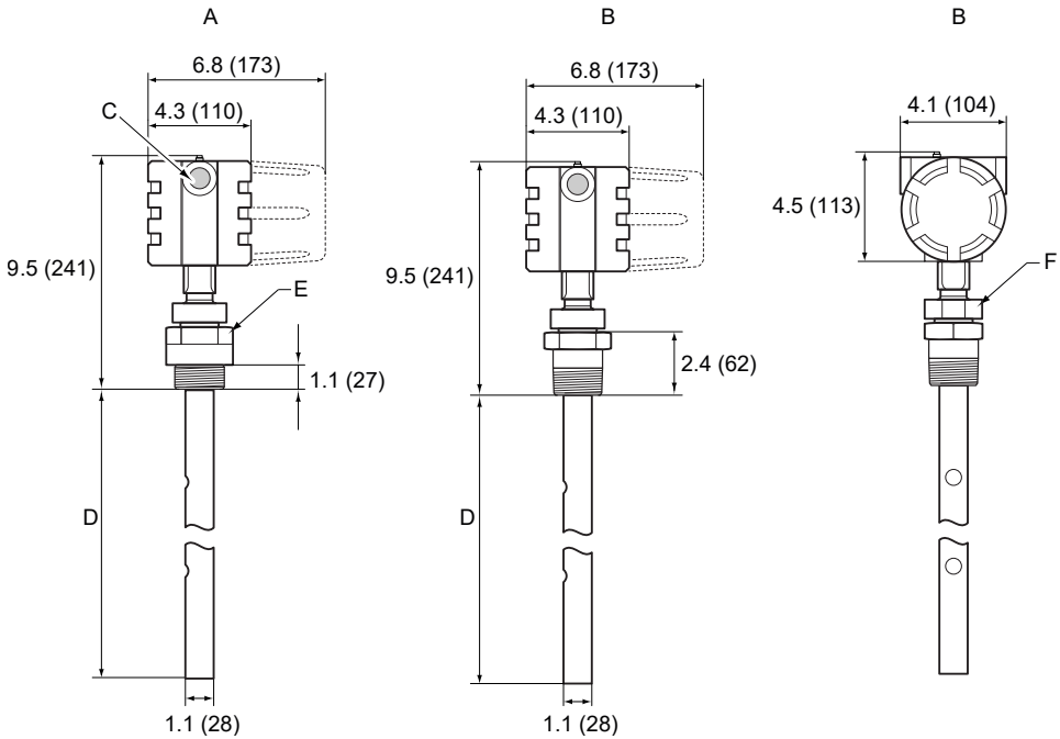
图 29: 采用螺纹连接的同轴导波杆
