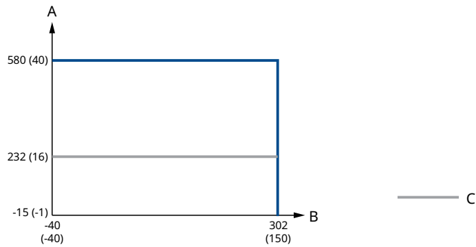
图 9: 最高额定值，标准储罐连接
