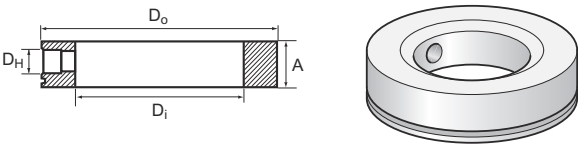
图 34: 冲洗连接环
