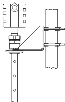
图 19: 露天应用中的同轴导波杆
