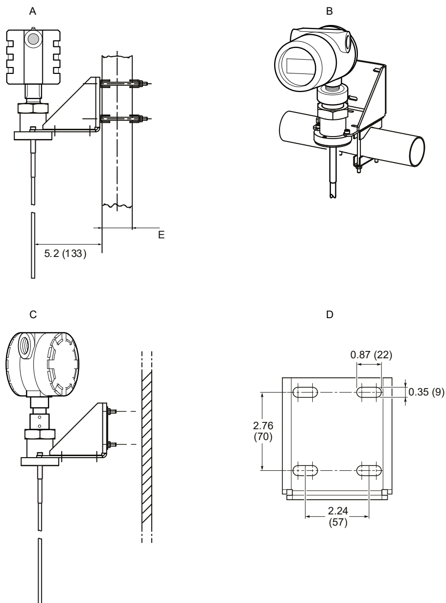
图 30: 支架安装
