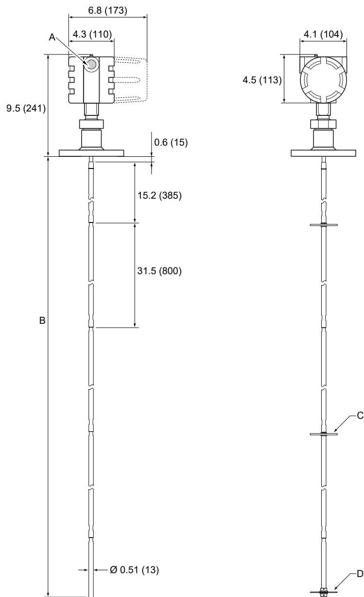
图 24: 采用法兰连接的分段硬单杆导波杆
