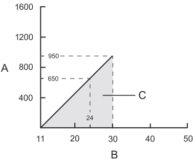
图 6: 本安安装
