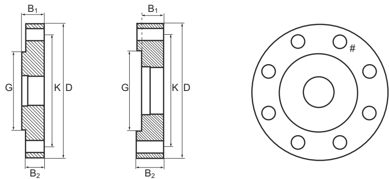
图 33: 专用法兰
