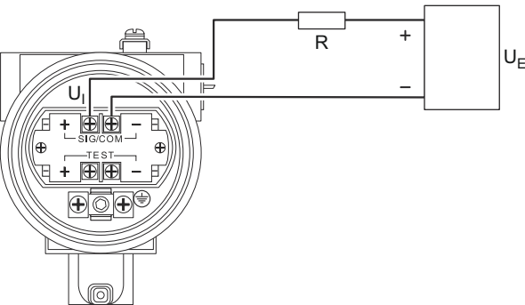
图 4: 用于 HART 的外部电源
