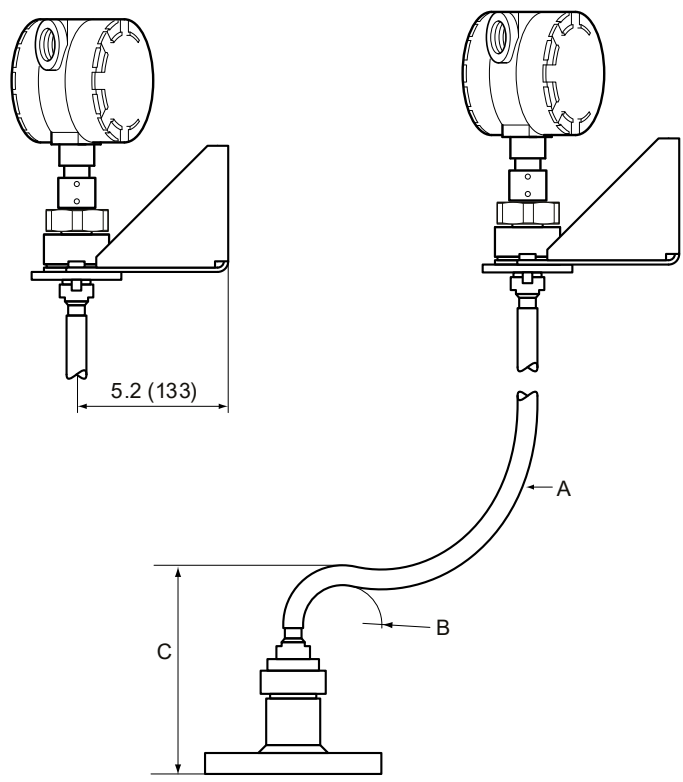
图 31: 延伸连接外壳
