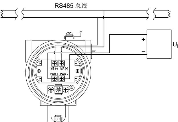
图 8: 用于 Modbus 的外部电源
