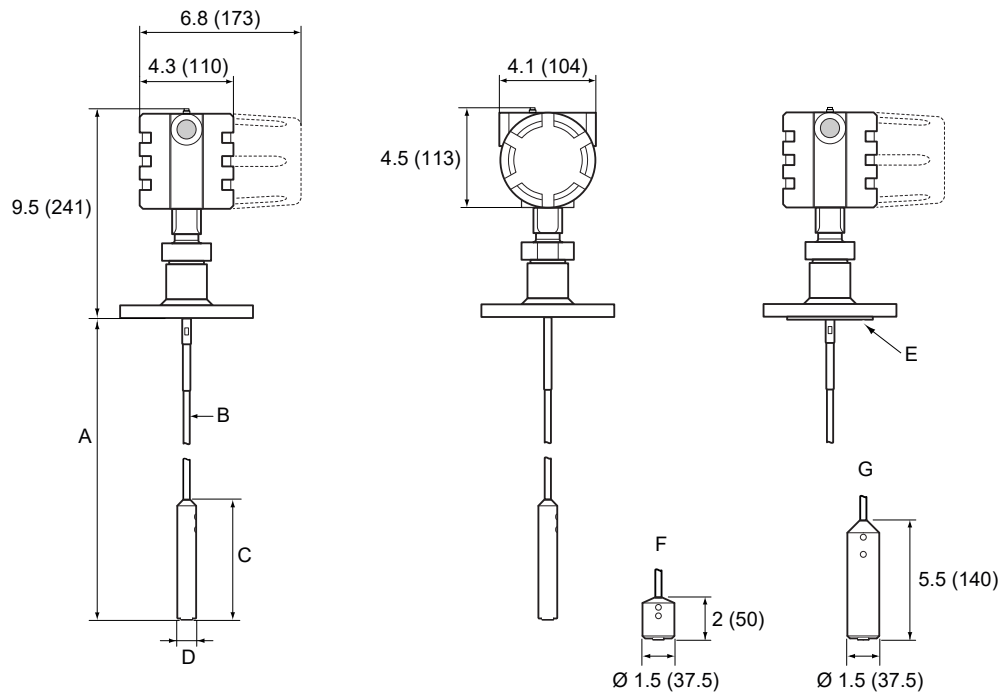
图 26: 采用法兰连接的软单杆导波杆
